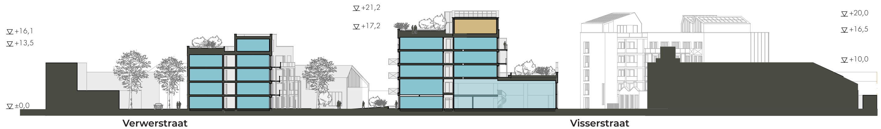
profiel A
